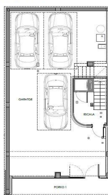
PLANTA SEMISOTERRANI
