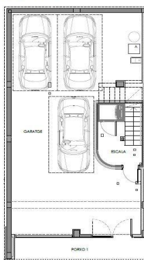
PLANTA SEMISOTERRANI
