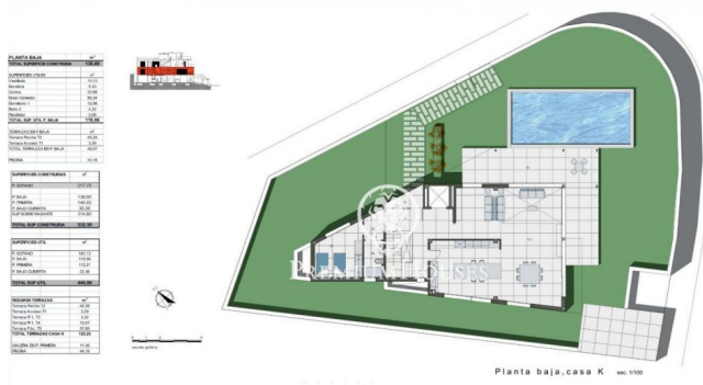
Planta baja, casa K
