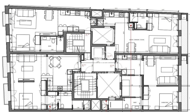
PLANTA SEGUNDA
